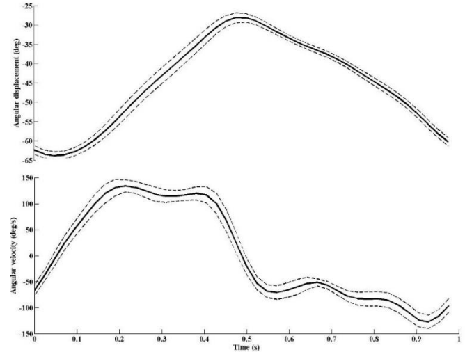
نمودار ۱: میانگین کل جابجایی و سرعت زاویه ای مفصل ران در سی سی سیکل رکاب زدن
